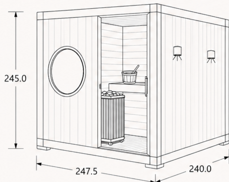
VISTA PERSPECTIVA (ISOMÉTRICA)
